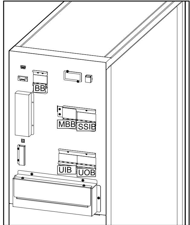
Vista posterior del SAI de 10-15 kVA con baterías internas
