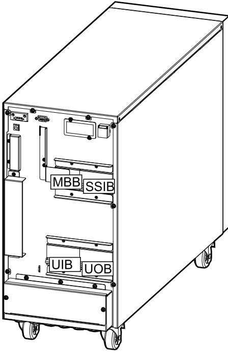
Vista posterior del SAI de 10-15 kVA con baterías externas
